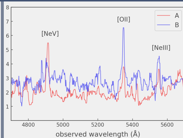
Keck-I
