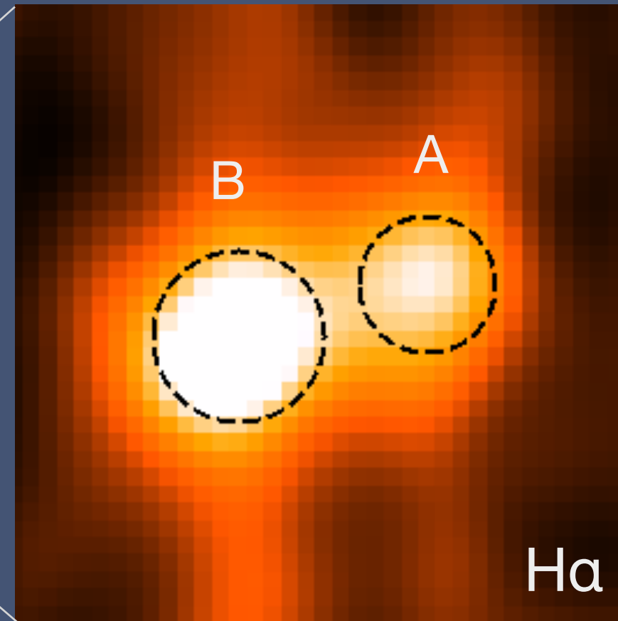
Gemini-N
