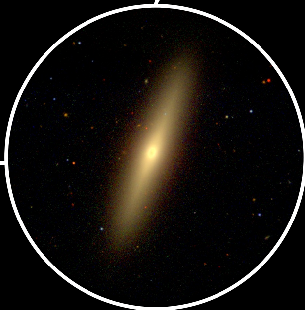
レンズ状銀河
